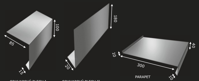
ODKVAPOVÝ PLECH I
