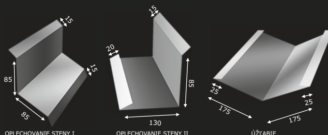
ÚPLECHOVANIE STENY I
