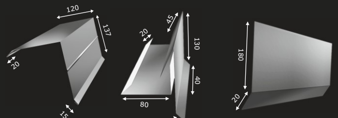
ZÁVETERNÁ LIŠTA I
