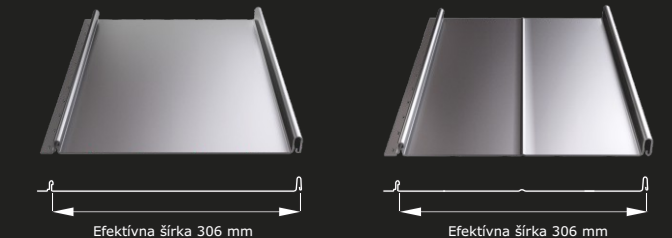
Efektívna šírka 306 mm
