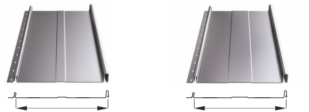
Efektívna šírka 205 mm
