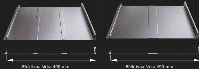
Efektívna šírka 490 mm
