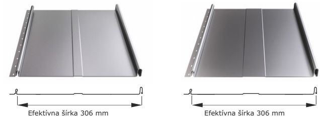
Efektívna šírka 306 mm
